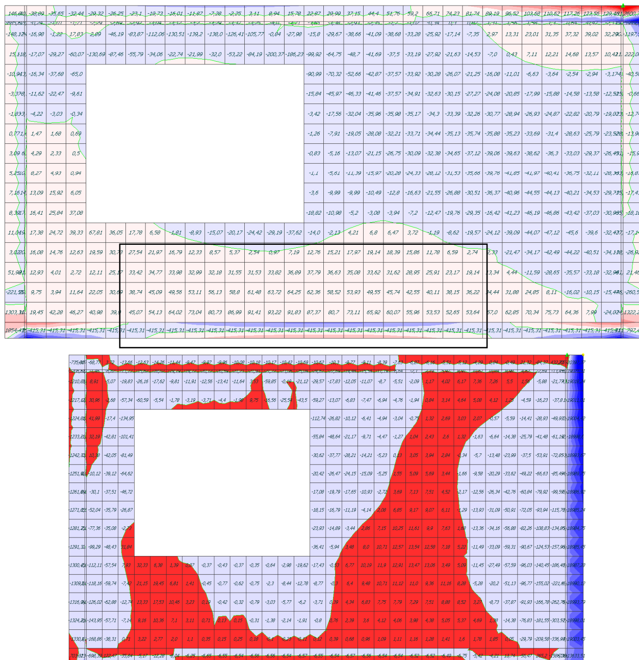
Рисунок П.Е.15 – Поля распределения напряжений \sigma_x (вверху) и \sigma_y (внизу) участка наружной поэтажно опертой стены, полученные по результатам расчета
